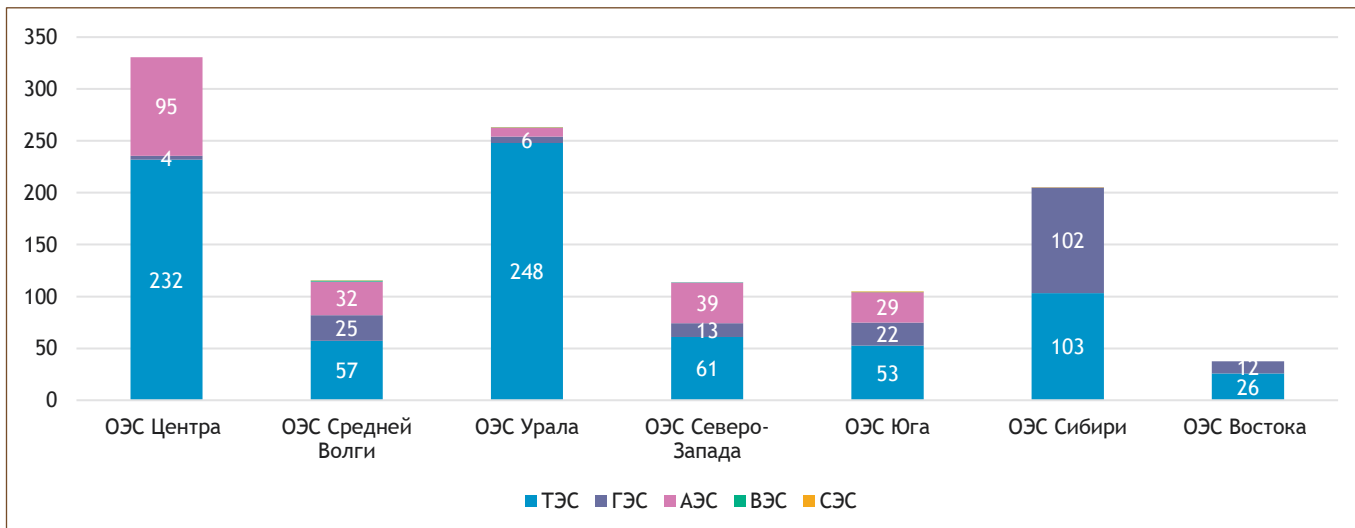
И. 3.12 Производство электроэнергии ОЭС по видам электростанций по итогам 2018 г, млн МВт
