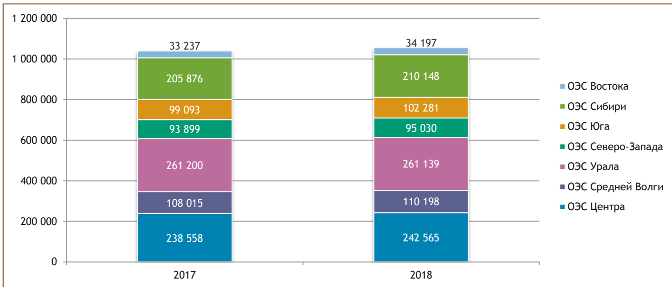
И. 3.16 Потребление электроэнергии по ОЭС России в 2017-2018 гг., тыс. МВт-ч
