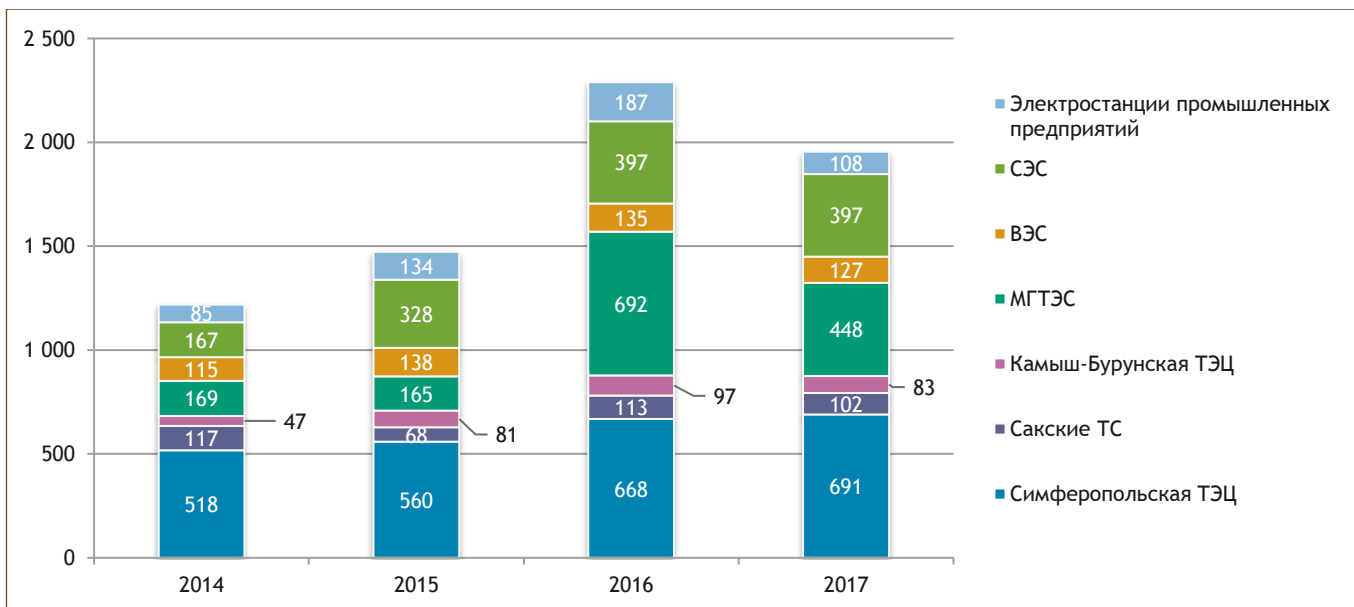
И. 3.14 Структура выработки электроэнергии электростанциями энергосистемы Республики Крым за период 2014 - 2017 гг., тыс. МВт-ч
