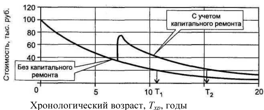
Рисунок. Зависимость стоимости оборудования от времени с учетом капитального ремонта
